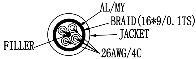
线材结构图
